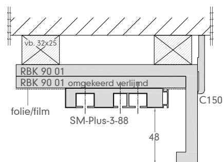
Plafondaansluiting (C150)
