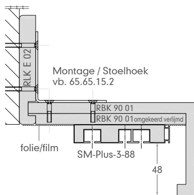
Muuraansluiting (RLK E 02)
