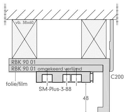
Plafondaansluiting (C200)
