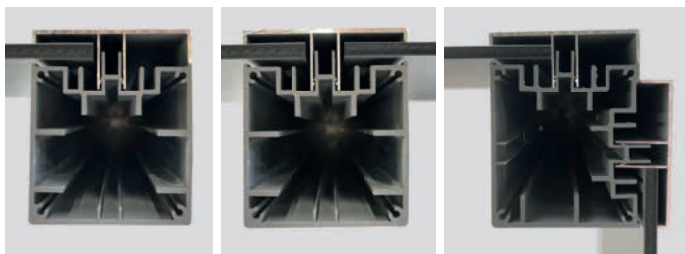
Poteau départ / finition
